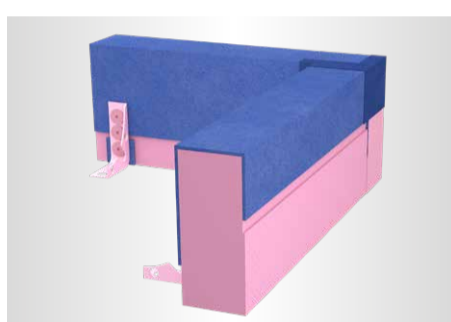
Bodenplattenschalung Thermo System Ecke FBV [ AUSSENECKE ]
