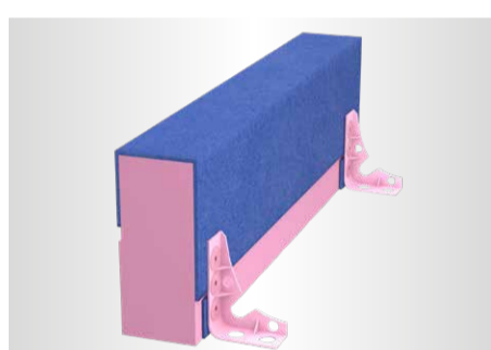
Bodenplattenschalung Thermo System Schenkel FBV [ MIT FRISCHBETONVERBUND- DICHTBAHN ]
