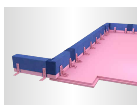
BODENPLATTE THERMO SYSTEM FBV [ MIT FRISCHBETONVERBUND-DICHTBAHN ]
